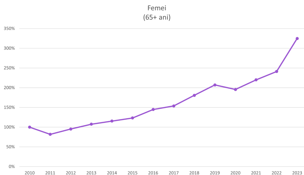
Fig. 14: Femei 65+, creștere procentuală (Grafic realizat în Excel)
