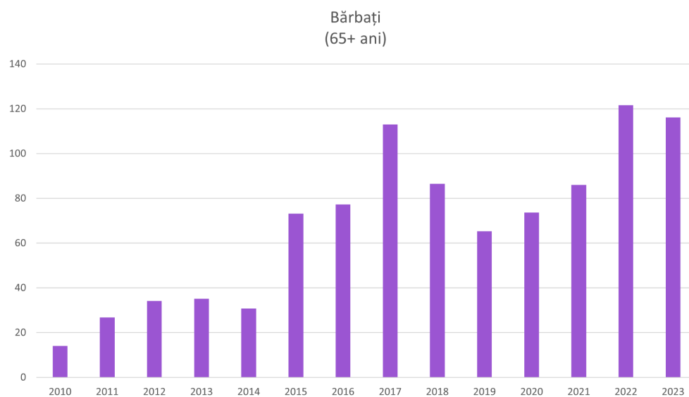
Fig. 17: Bărbați 65+, valori absolute (Grafic realizat în Excel)
