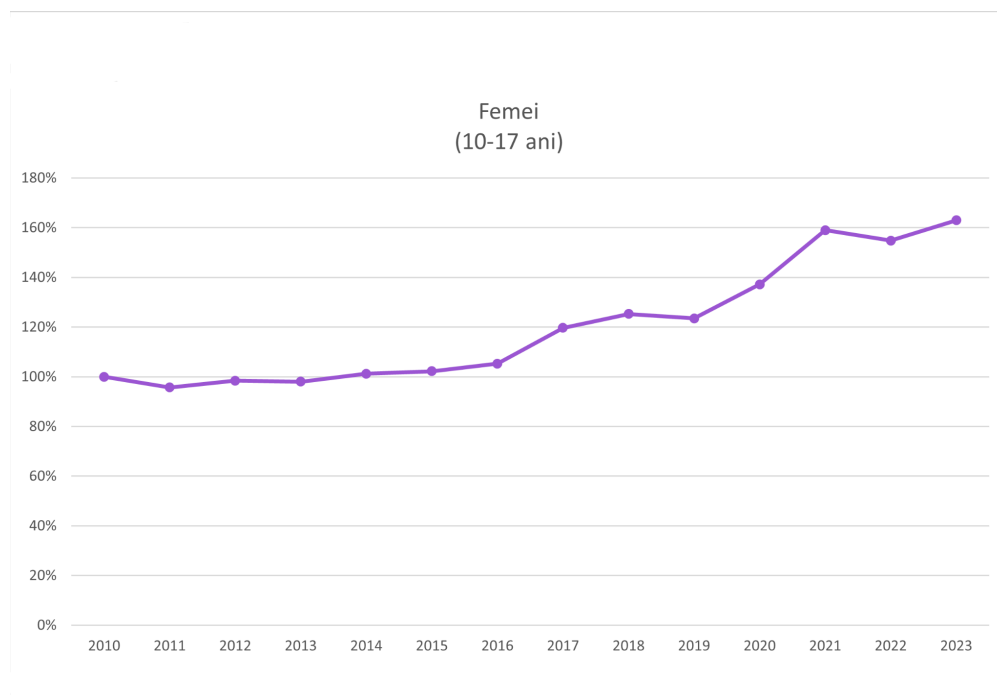
Fig. 12: Femei 10-17, creștere procentuală (Grafic realizat în Excel)
