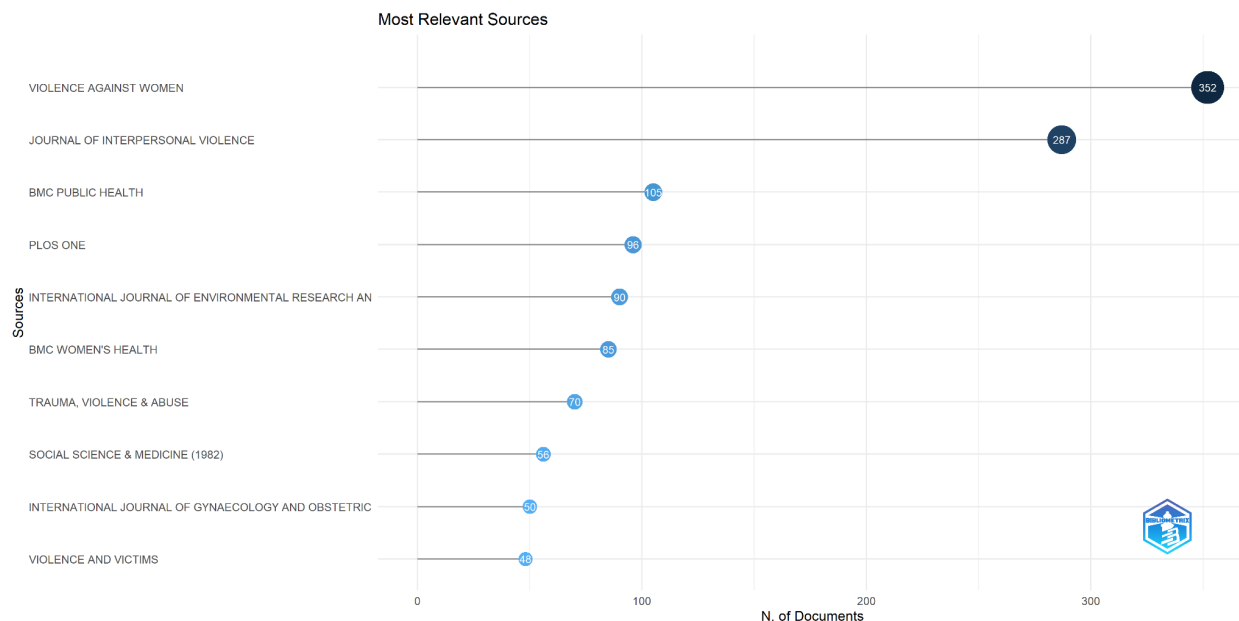
Fig. 7 : Topul surselor relevante pentru termenul violence against women (Grafic realizat în Biblioshiny )
