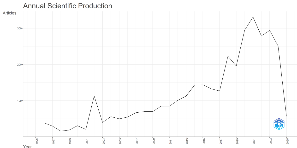
Fig. 4 : Evoluția generală a publicațiilor pentru termenul violence against women (Grafic realizat în Biblioshiny )
