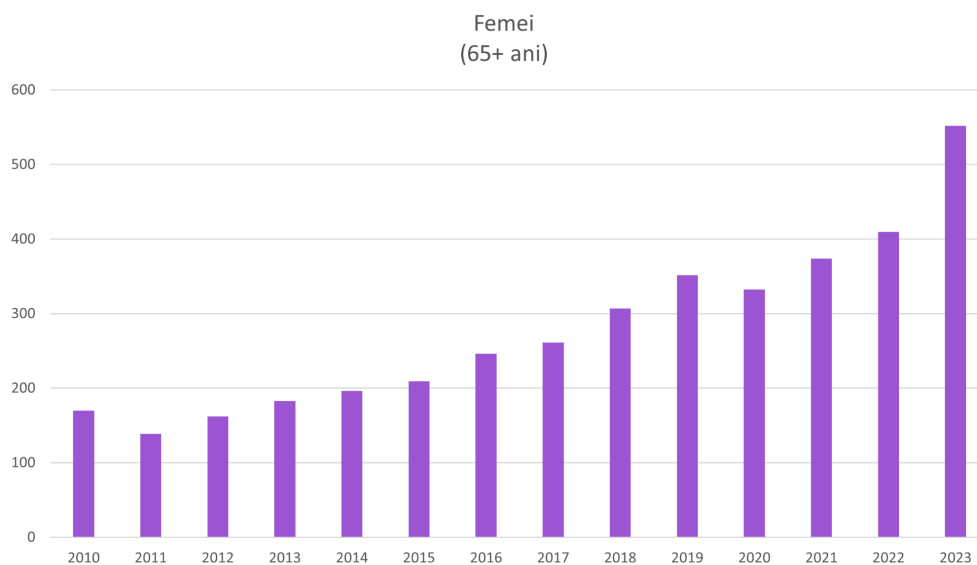
Fig. 13: Femei 65+, valori absolute (Grafic realizat în Excel)
