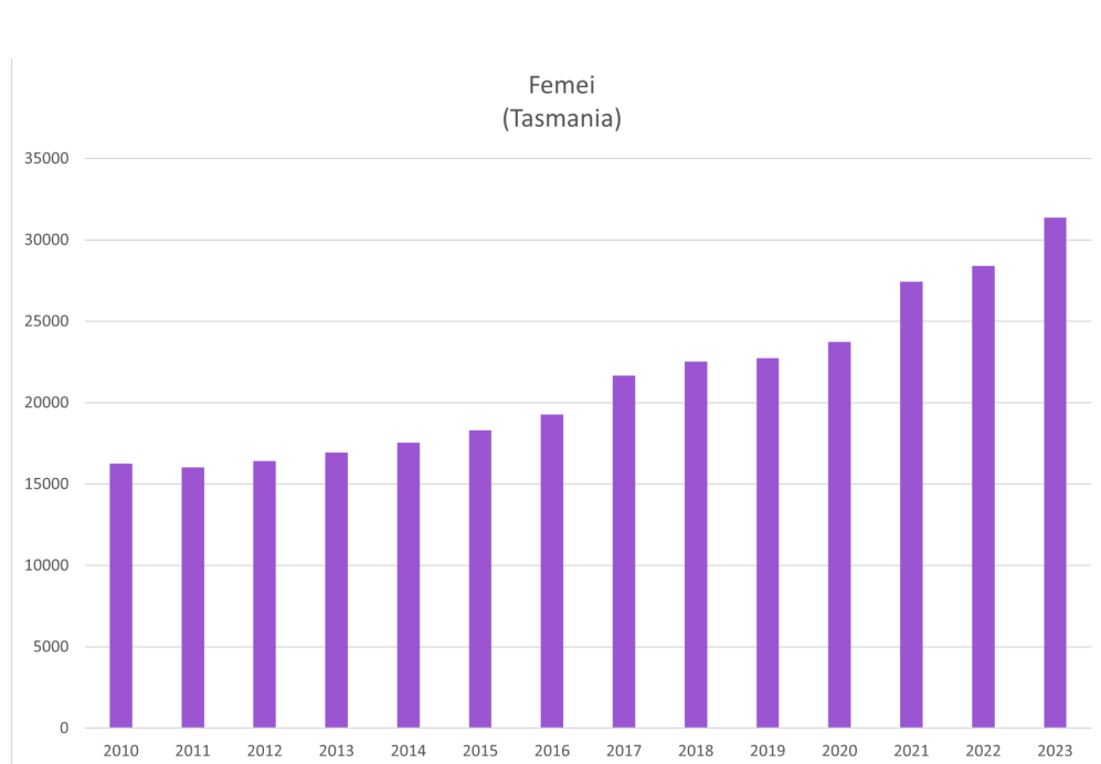
Fig. 22: Femei, Tasmania (Grafic realizat în Excel)
