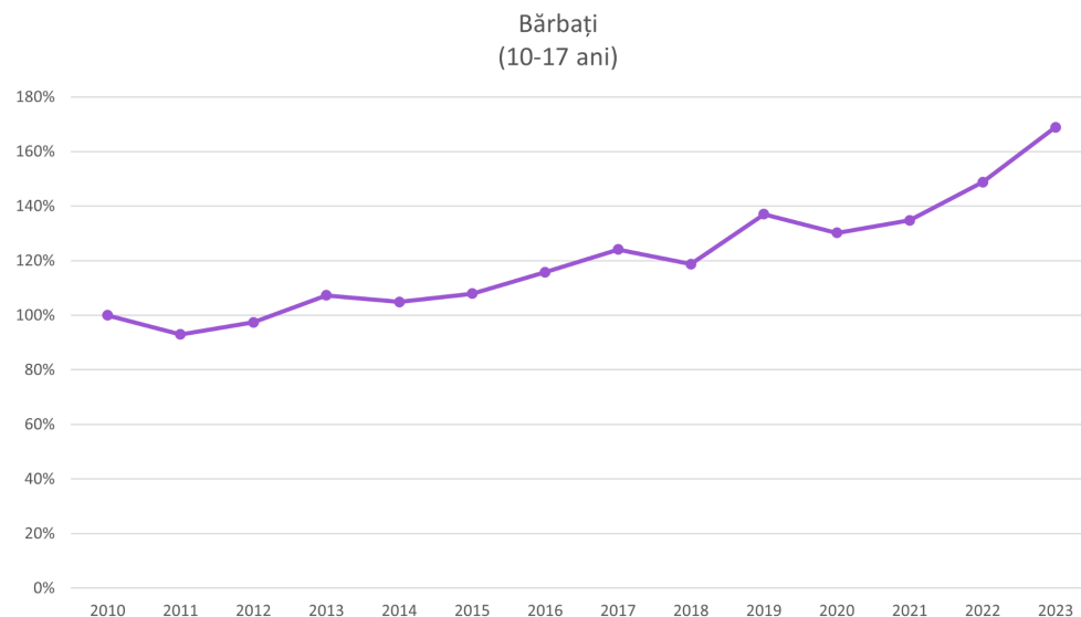
Fig. 16: Bărbați 10-17, creștere procentuală (Grafic realizat în Excel)
