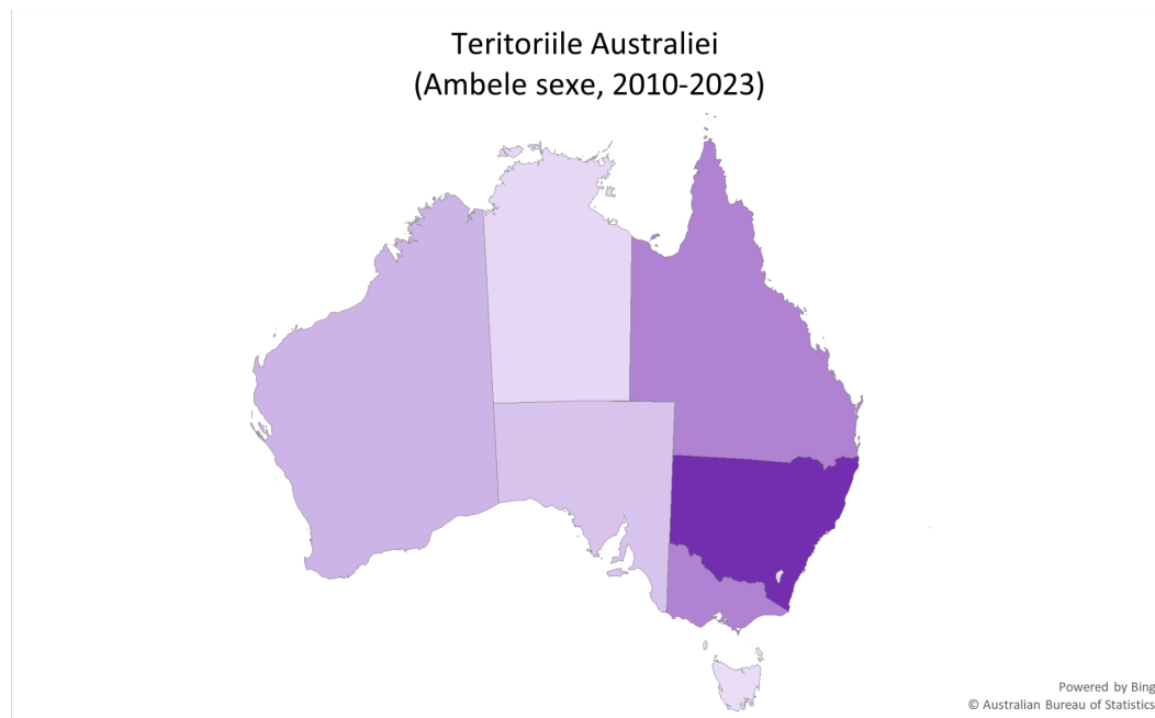
Fig. 24: Australia, harta continentului (Grafic realizat în Excel)
