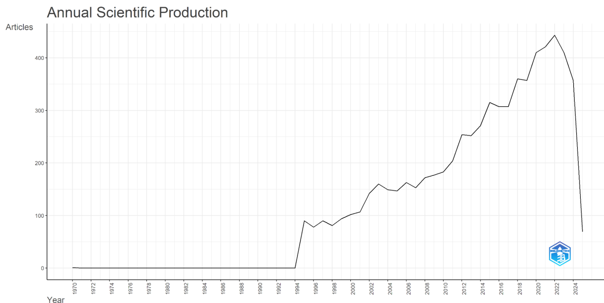
Fig. 3 : Evoluția generală a publicațiilor pentru termenul physical abuse (Grafic realizat în Biblioshiny )
