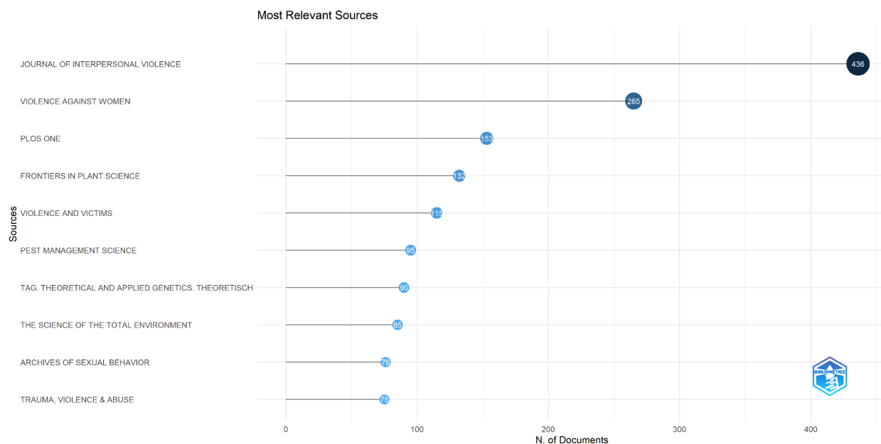
Fig. 5 : Topul surselor relevante pentru termenul rape (Grafic realizat în Biblioshiny )
