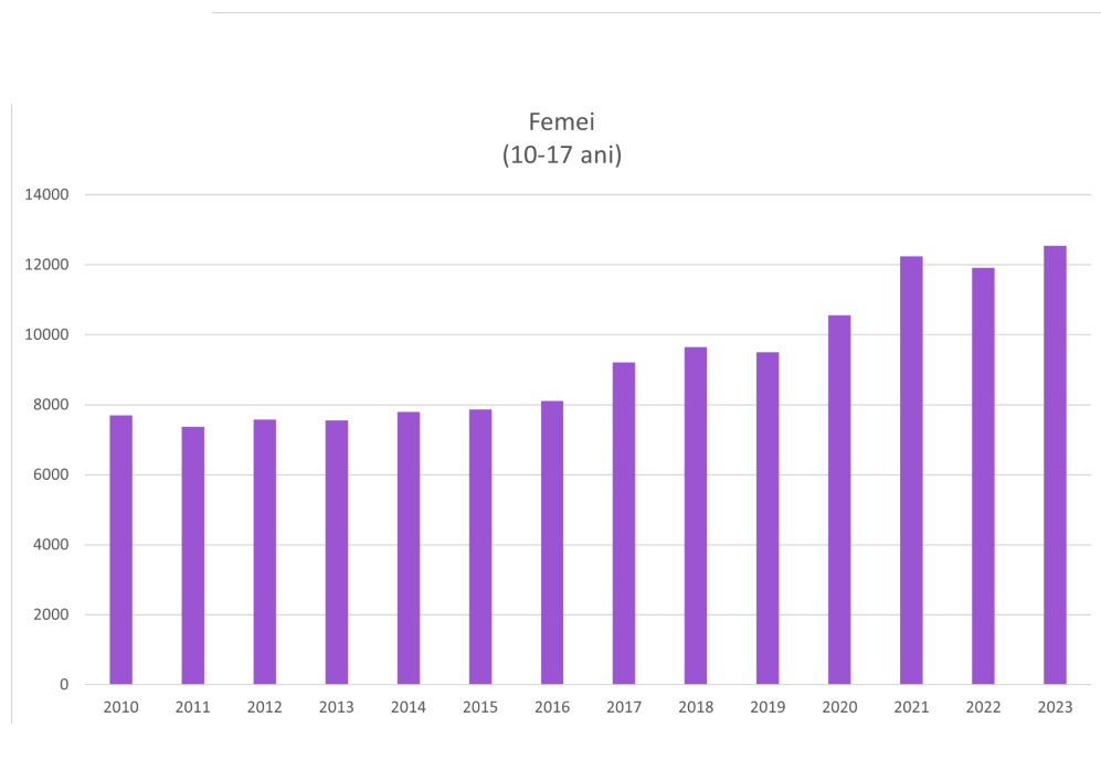
Fig. 11: Femei 10-17, valori absolute (Grafic realizat în Excel)
