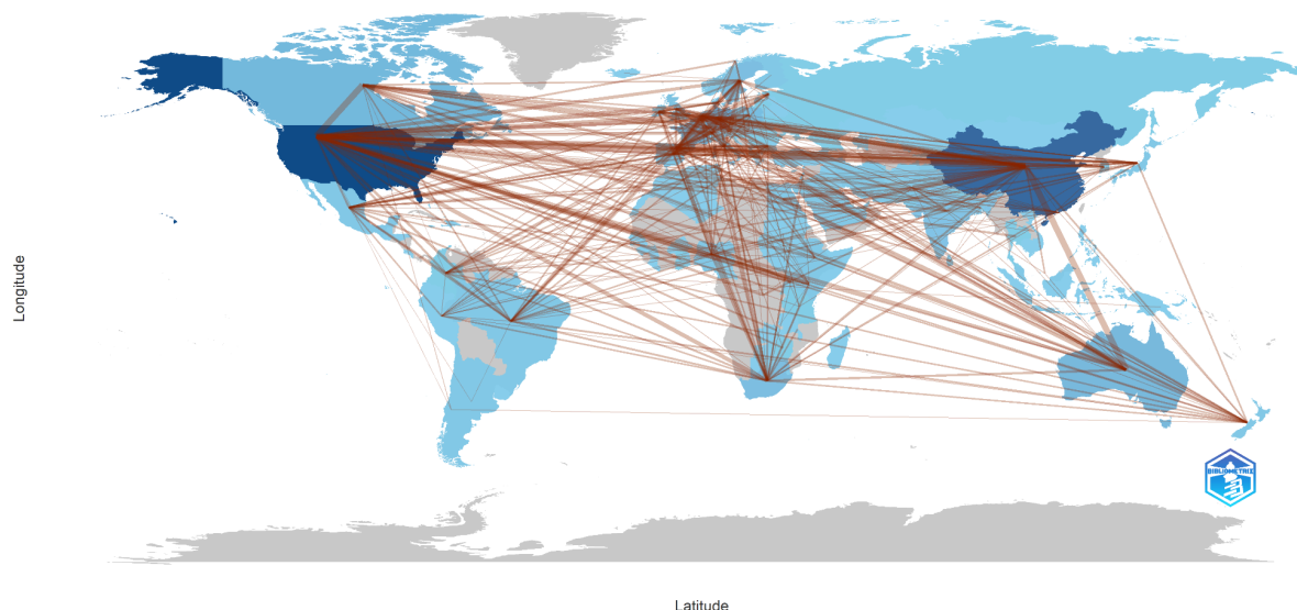
Fig. 8 : Harta colaborărilor internaționale în cercetarea privind termenul rape (Grafic realizat în Biblioshiny )
