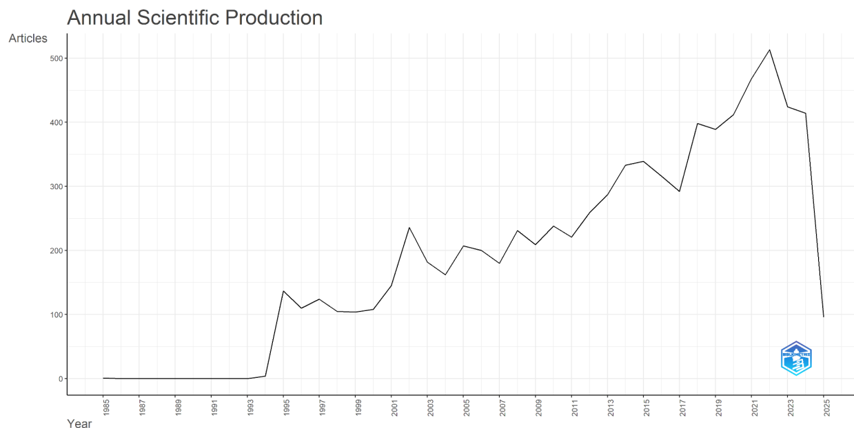
Fig. 2 : Evoluția generală a publicațiilor pentru termenul rape (Grafic realizat în Biblioshiny )
